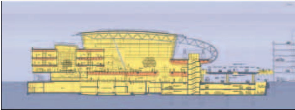
Querschnitt Zentralgebäude
