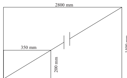
Pilkington Szkło z Sitodrukiem Minimalne i maksymalne wymiary szyby pokrywanej sitodrukiem
