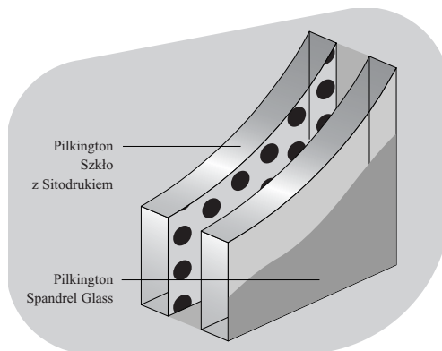
Montaż szyby zespolonej na fasadzie bez wentylacji: szyba zewnętrzna – Pilkington Szkło z Sitodrukiem, szyba wewnętrzna – Pilkington Spandrel Glass
