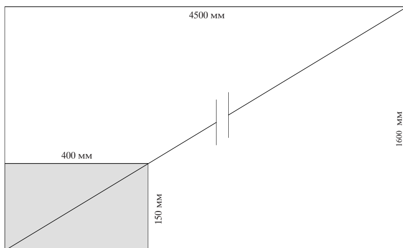
Минимальные и максимальные размеры стекла Pilkington Spandrel Glass
