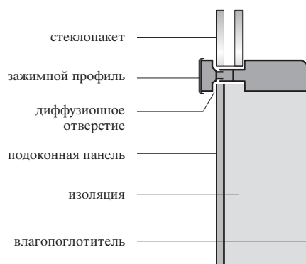
Без вентиляционного зазора
