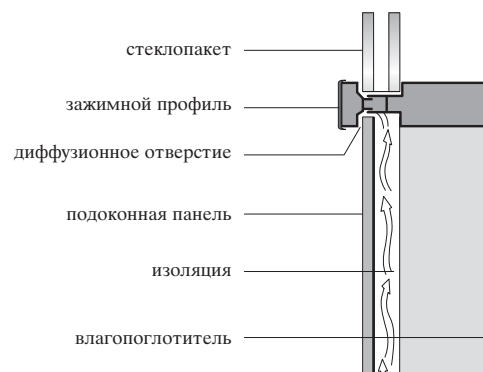
С вентиляционным зазором
