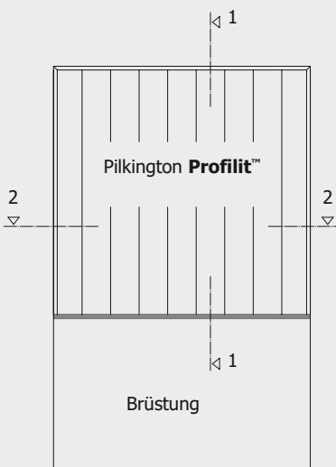
Ansicht
