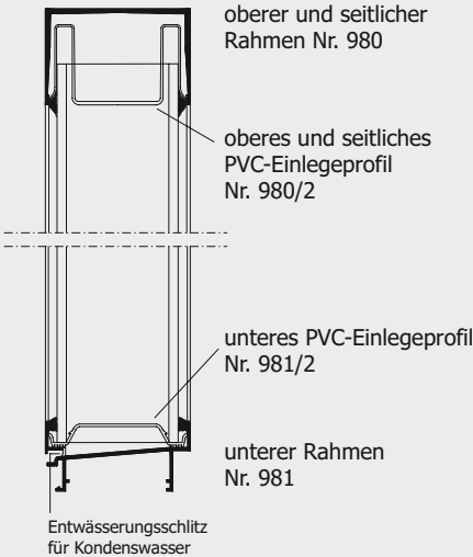
Vertikalschnitt 1-1
