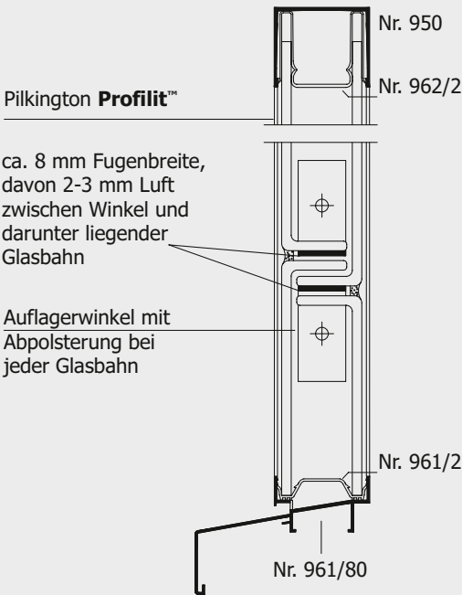
Schnitt 1-1
