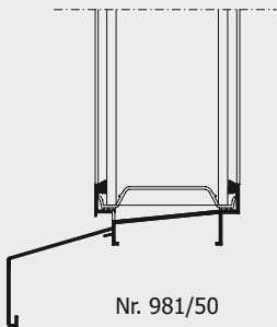
Horizontalschnitt 2-2
