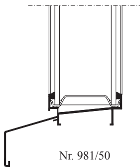
Horizontalschnitt 2-2
