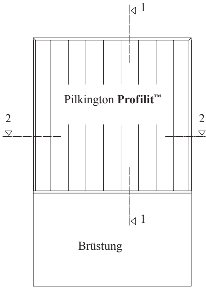
Ansicht
