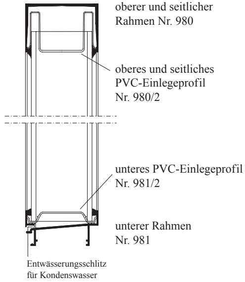
Vertikalschnitt 1-1
