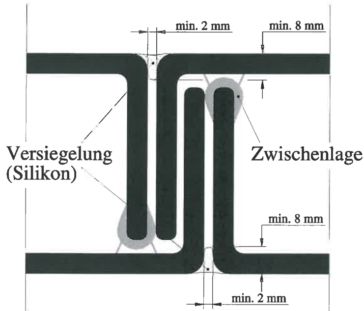
Zeichnung 2: Fugenausbildung bei einschaliger Pilkington Profilit™ - Verglasung:
