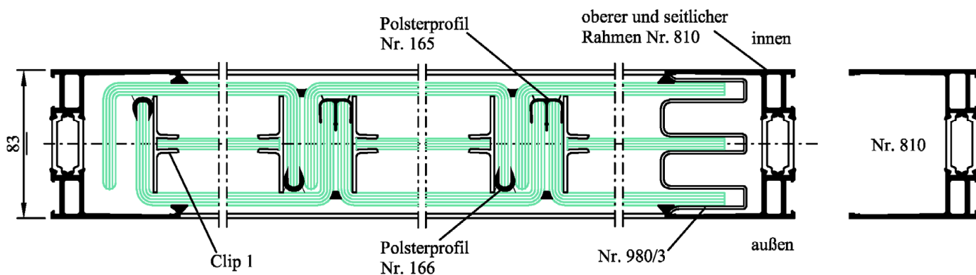
Horizontalschnitt 2-2
