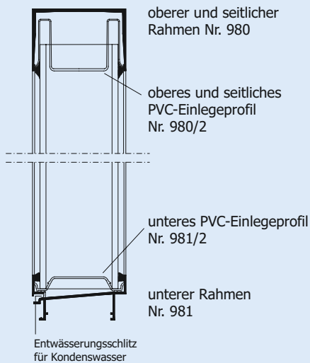
Vertikalschnitt 1-1
