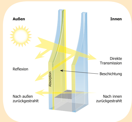
Isolierglaseinheit mit beschichtetem Sonnenschutzglas
