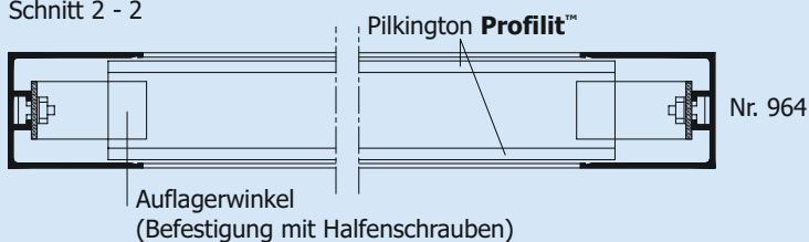
Schnitt 2 - 2
