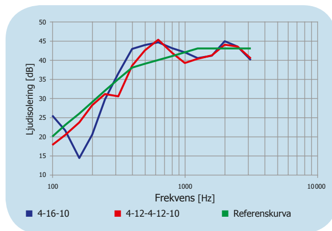
Figur 5: Jämförelse mellan två isolerglas med olika uppbyggnad där R_w = 39 dB
