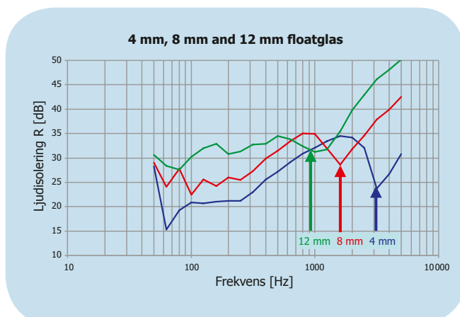
Figur 6: Glastjocklekens inverkan på koincidensfrekvens
