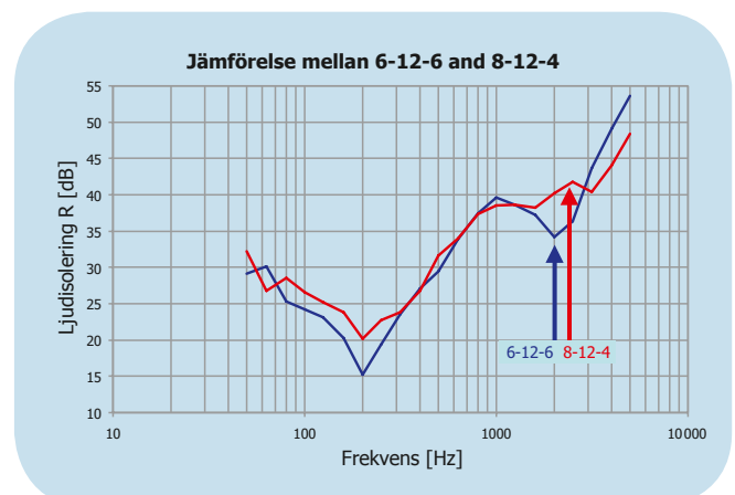
Figur 7: Asymmetrisk glasuppbyggnad för att minska koincidens
