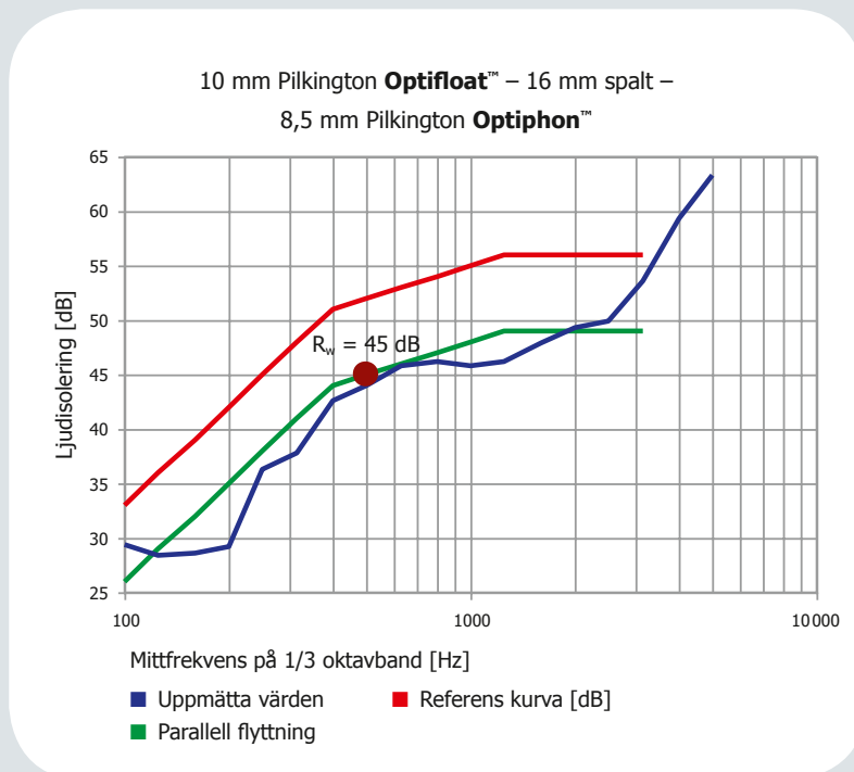
Figur 4: Bestämning av ljudisoleringsvärdet R_w
