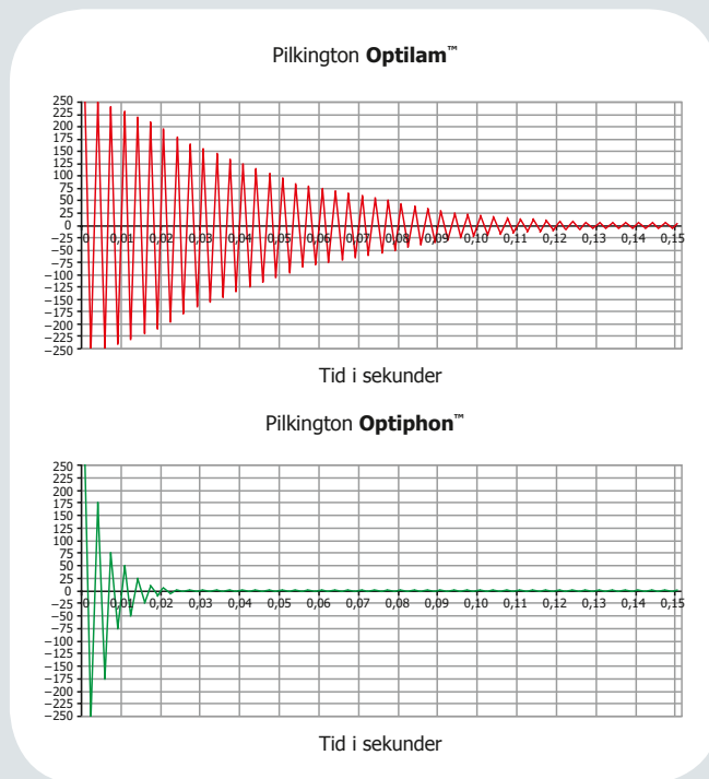
Figur 9: Illustrationen visar den imponerande skillnaden mellan Pilkington Optilam™ och Pilkington Optiphon™ ur ljudteknisk synvinkel.
